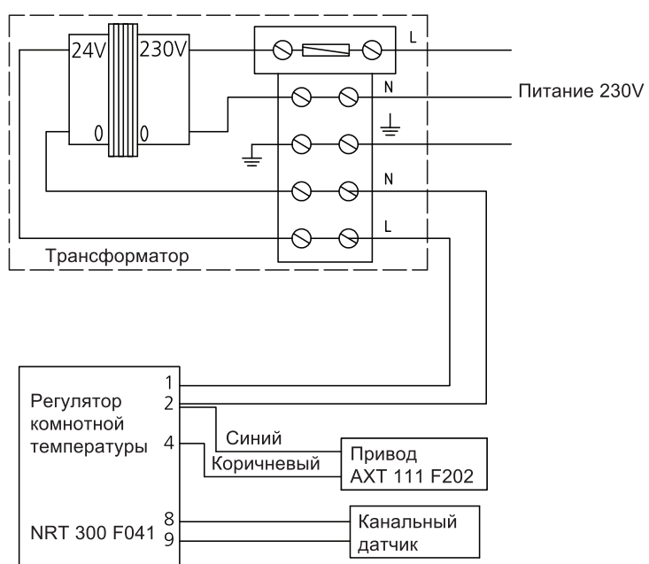
Схема электропроводки
